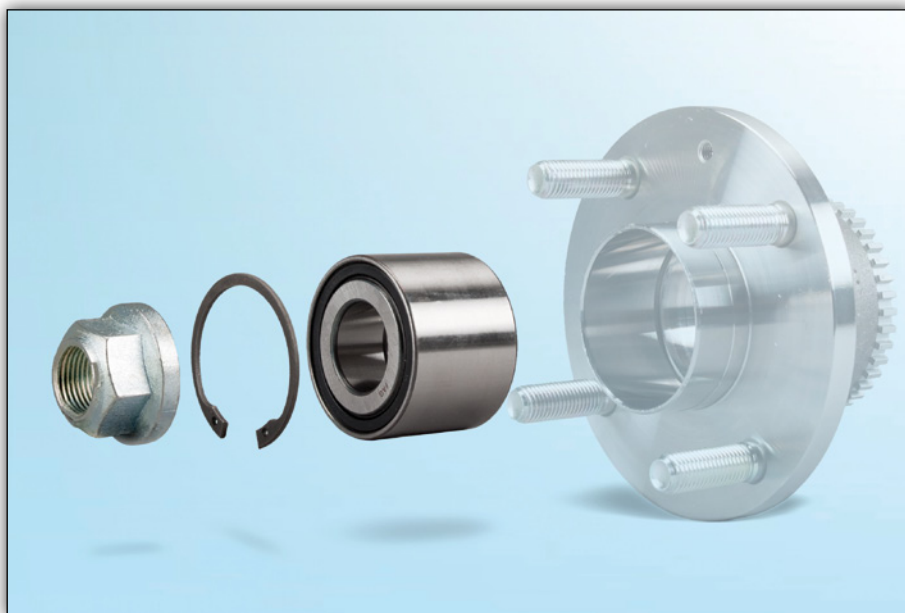
Bild 1: Das FAG-Radlager-KIT 713 6448 00 als Reparaturlösung - die Radnabe muss hierbei nicht ersetzt werden.
