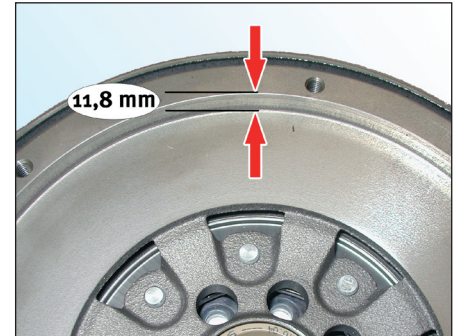
Bild 2: 415 0239 10 / 415 0243 10 (neue ZMS-Version)
