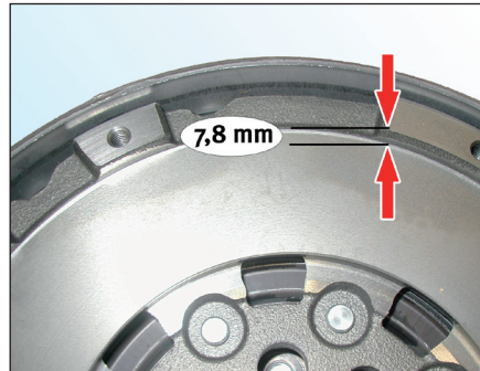
Bild 1: 415 0148 10 / 415 0151 10 (alte ZMS-Version)
