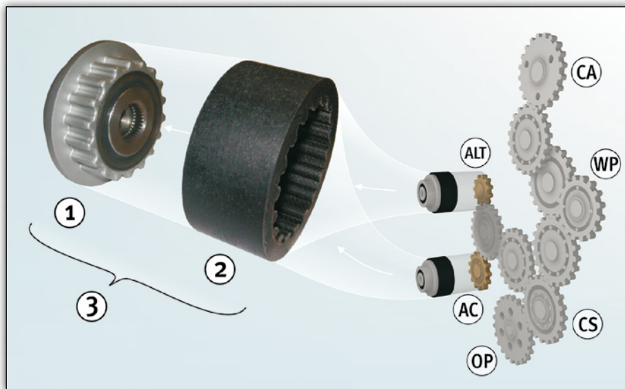
Bild 1: Generatorenfreilauf mit flexibler Kupplungsmuffe und Stirnradtrieb
