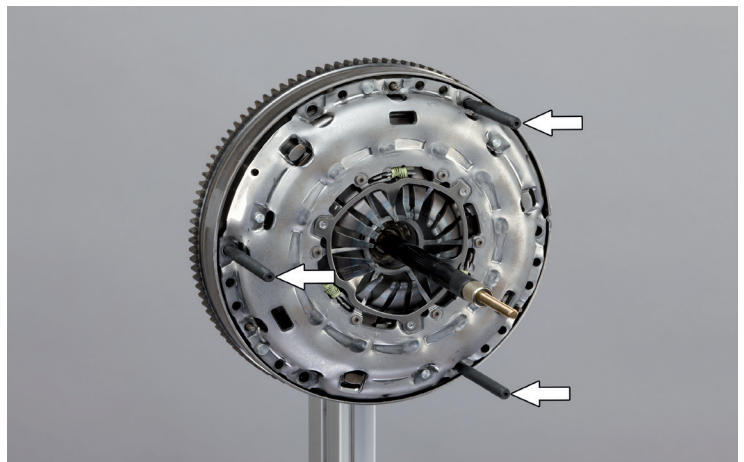
Bild 2: Stehbolzen zur Aufnahme des Spindelträgers
