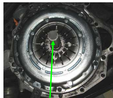
Zentrierwerkzeug
