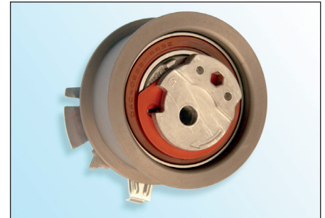
Bild 2: 531 0628 30 (neue Ausführung)
