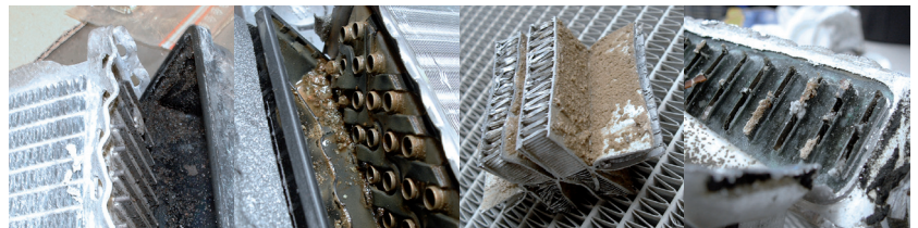
Abbildung 2: Ablagerungen wie Rost, Kalk, Dichtmittel oder andere Fremdkörper sorgen für Blockaden und reduzieren die Kühlleistung
