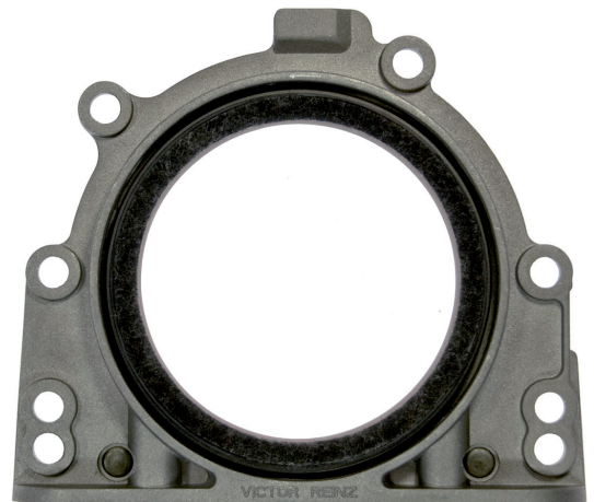
Abbildung 1_Integrierter Wellendichtring 81-90006-00
