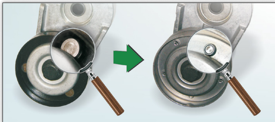
Bild 1: Detailansicht der Laufrollen in der bisherigen Ausführung (links) und der neuen Ausführung (rechts)
